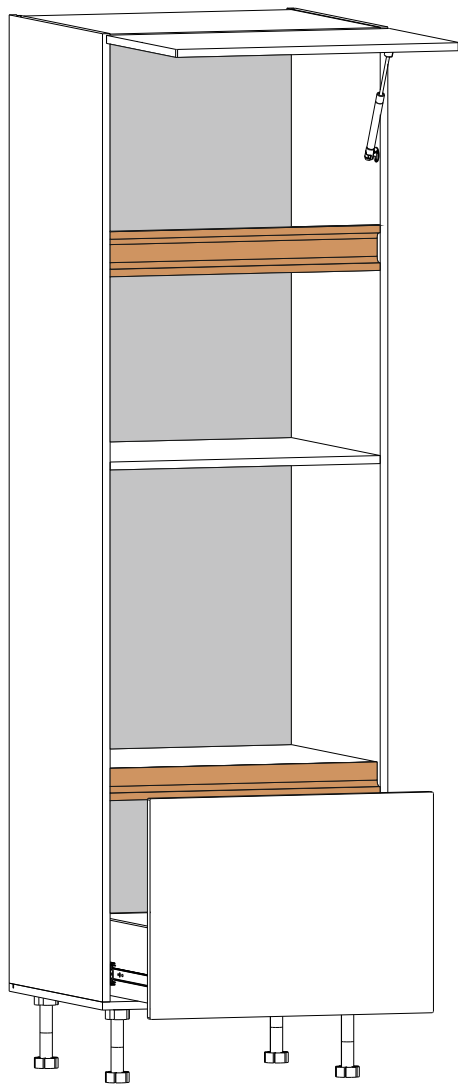
Пенал П-1н (600*586*2096)
